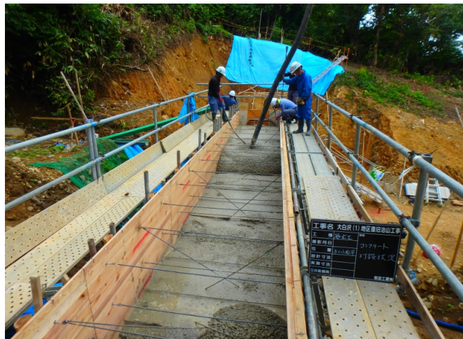
木製残存型枠（施工状況）
